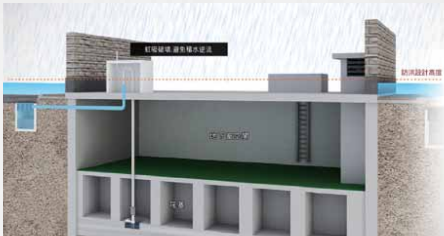
<虹吸破壞裝置>
